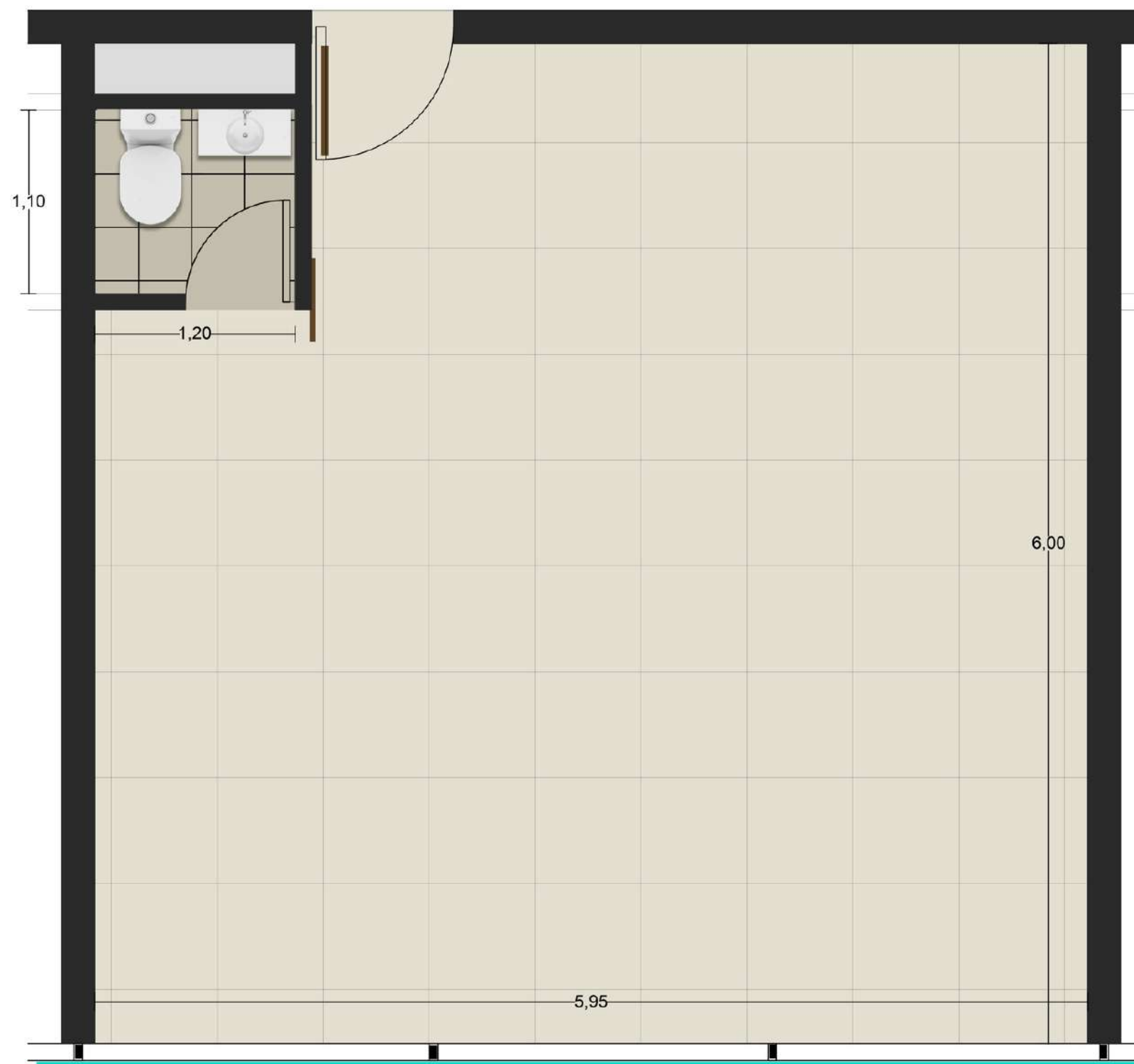
PLANTA TIPO SUPERFICIE 39.69 M2 - OF. 19
